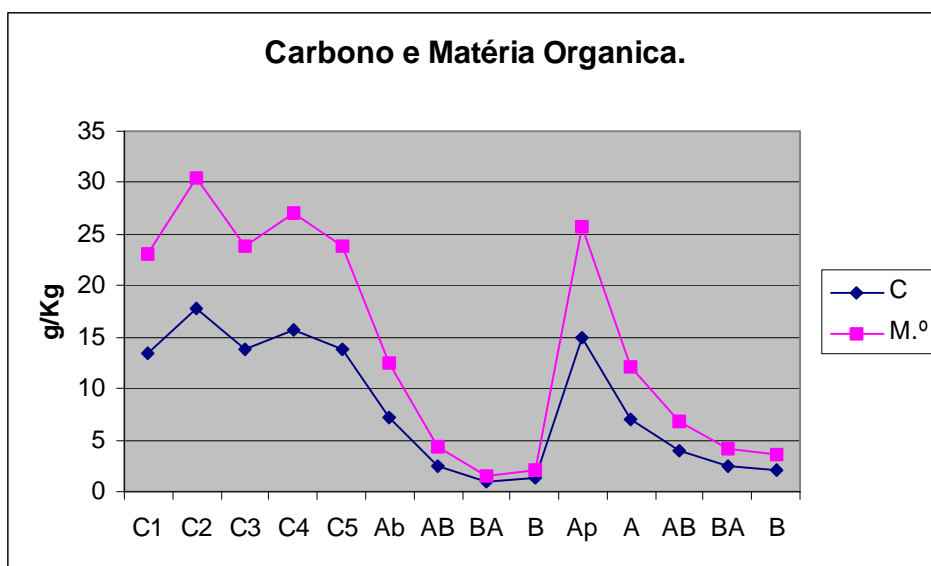
Gráfico 46. Distribuição de Carbono e Matéria Orgânica.
